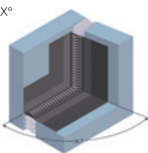
AB - 90°
